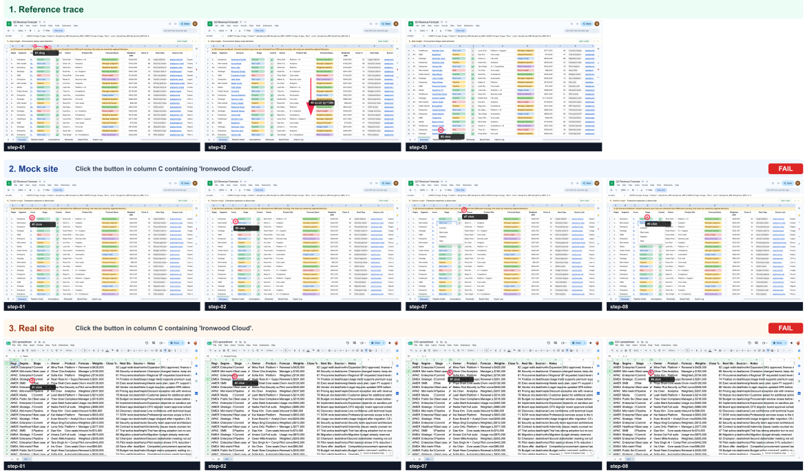
(b) Qwen3-VL
